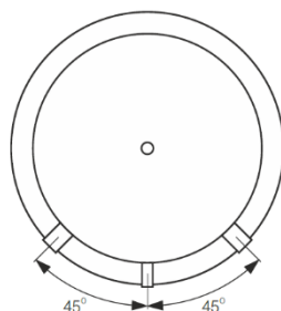
SV/SVW 200-500 I
