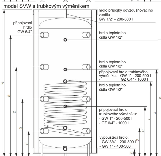
SV/SVW 200-500 I
